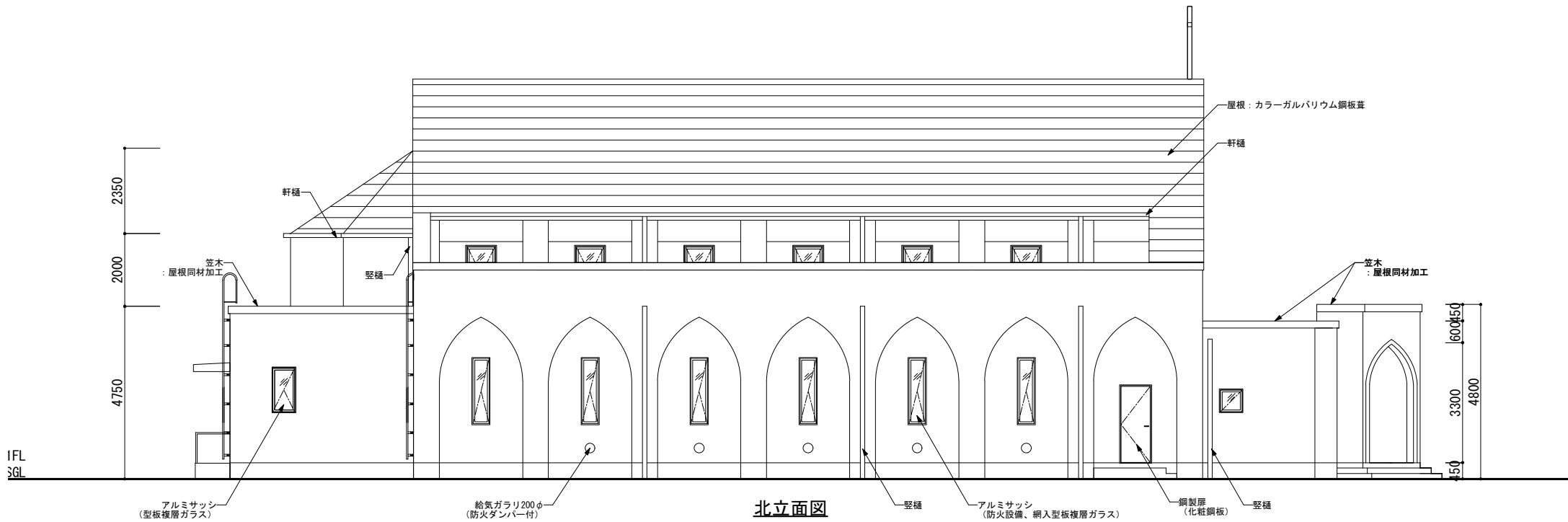
南立面図
